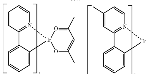
Ir(ppy) 2 (acac)
