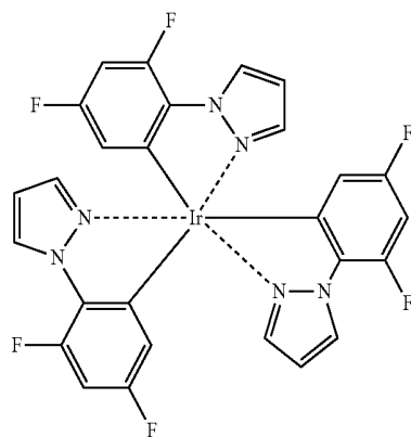
Ir(dfppz) 3
